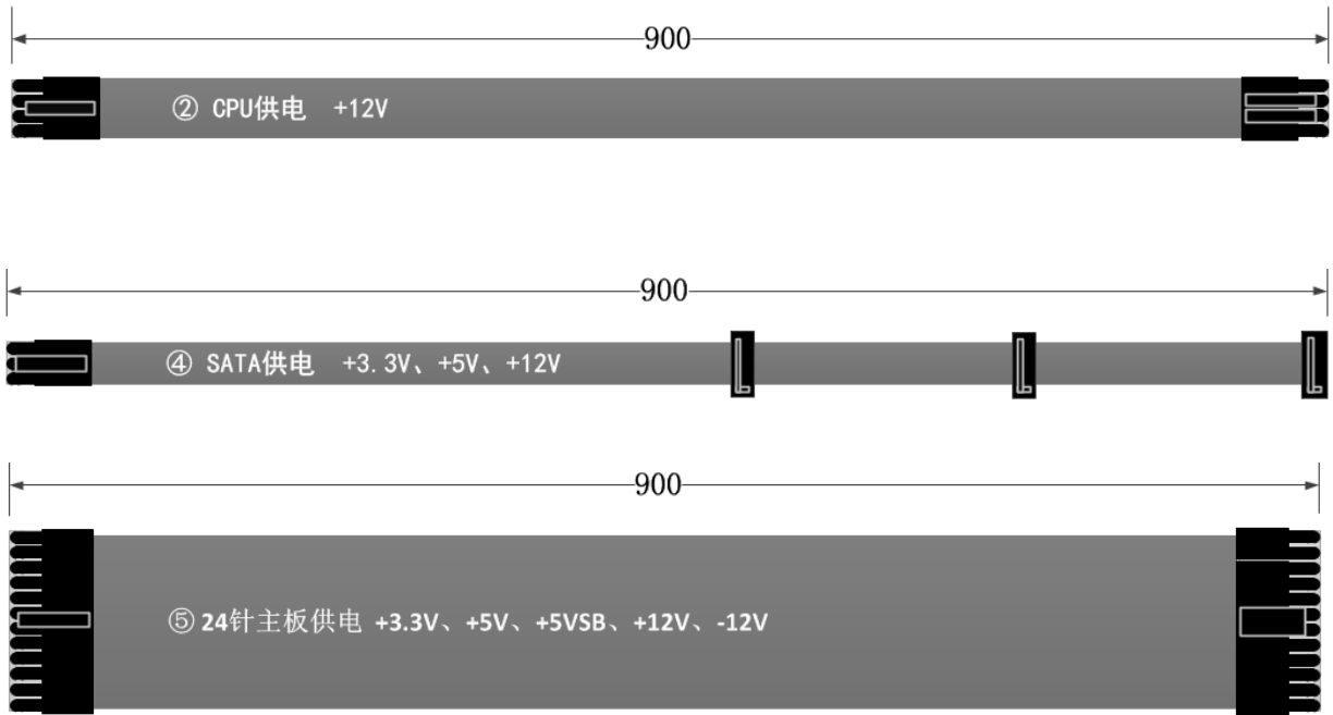
图12 900mm实训专用加长线束
